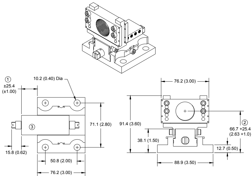
Figure 19 330850 DIN Mount 3300 XL 25 mm ProximitoR® Sensor
