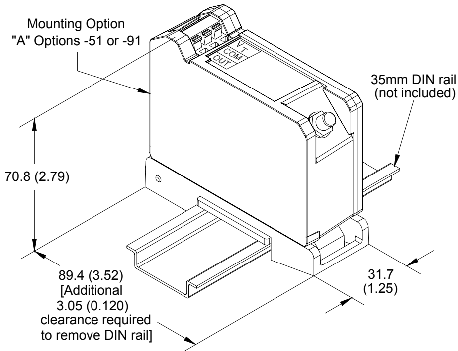
Figure 19 330850 DIN Mount 3300 XL 25 mm ProximitoR® Sensor
